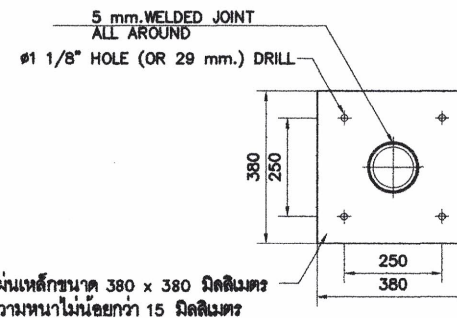
รายละเอียด แผ่นเหล็ก
