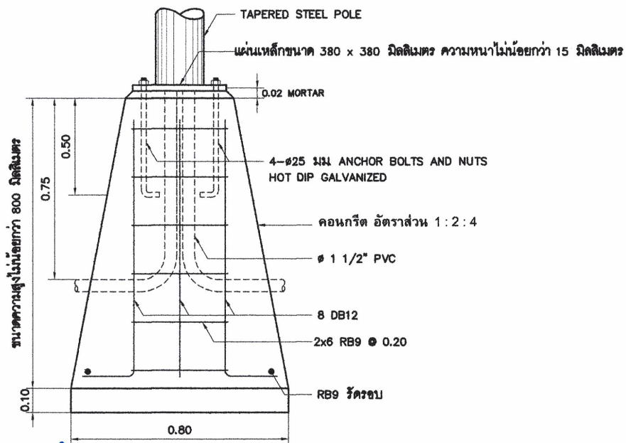
แบบขยายด้านข้าง
